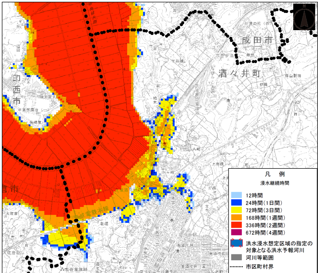
図表 21 利根川水系利根川洪水浸水想定区域図（浸水継続時間）
