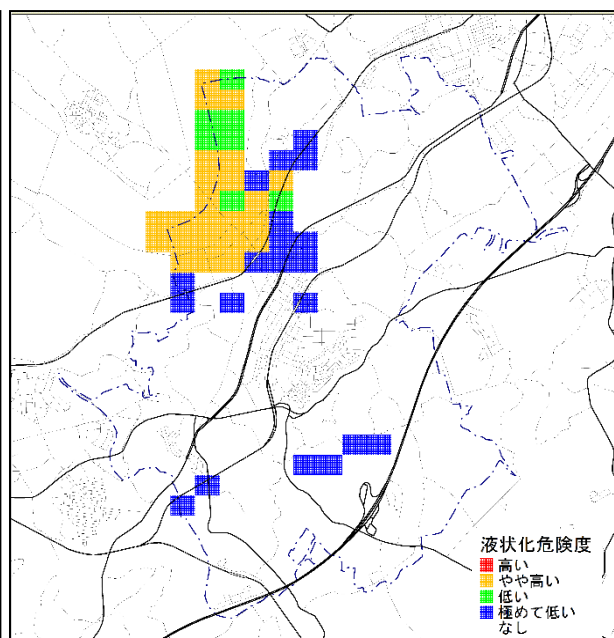
図表 16 液状化危険度予測図
