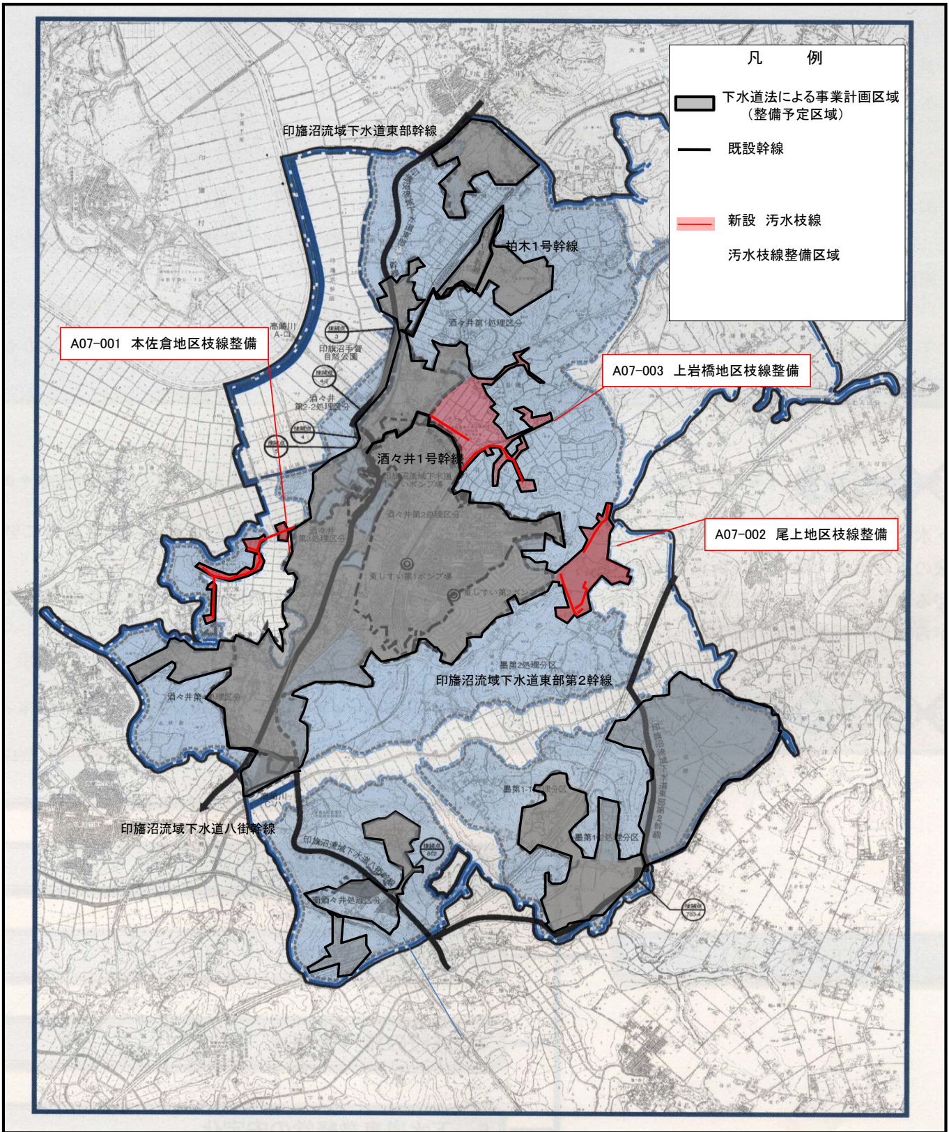
印旛処理区計画図
